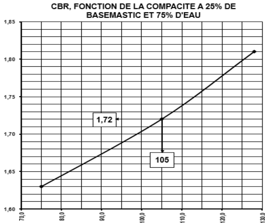
Figure 9 : Courbe de l'évolution du CBR avec le dosage au basemastic à 25%
