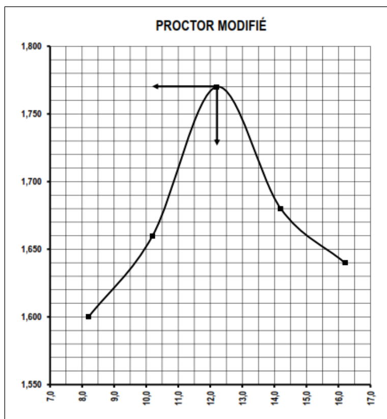
Figure 4 : Courbe Proctor Modifié du sol phosphaté traité au basemastic (35% de basemastic et 65% d'eau)
