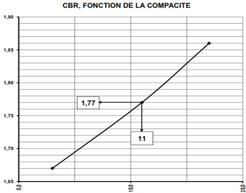
Figure 8 : Courbe CBR du sol phosphaté cru
