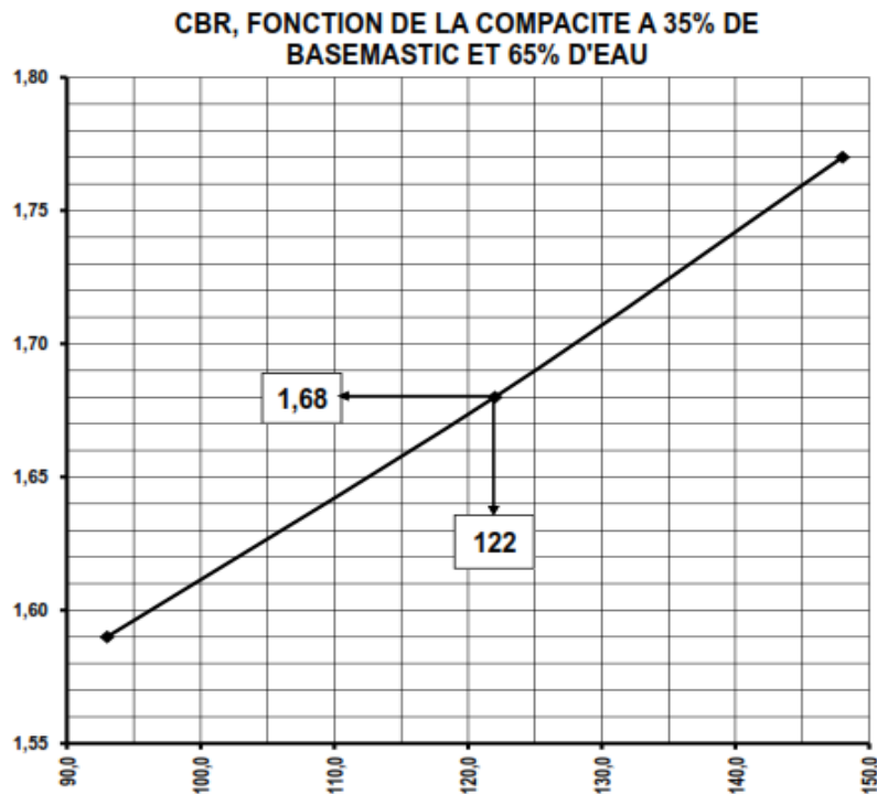
Figure 10 : Courbe de l'évolution du CBR avec le dosage au basemastic à 35%
