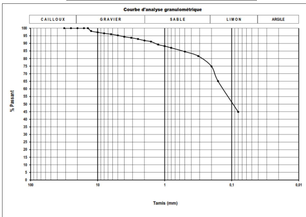
Figure 2 : Courbe d'analyse granulométrique du résidu de phosphate de Kpémé
