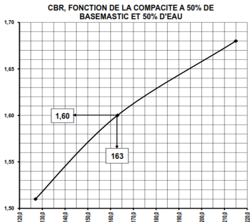
Figure 11 : Courbe de l'évolution du CBR avec le dosage au basemastic à 50%
